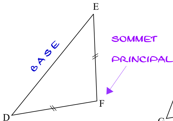
DEF est un triangle
