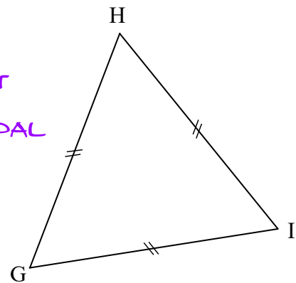
GHI est un triangle
