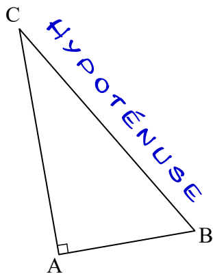
ABC est un triangle
